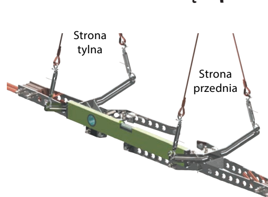
Ustawienie kąta pochylenia wzdłużnego \beta
