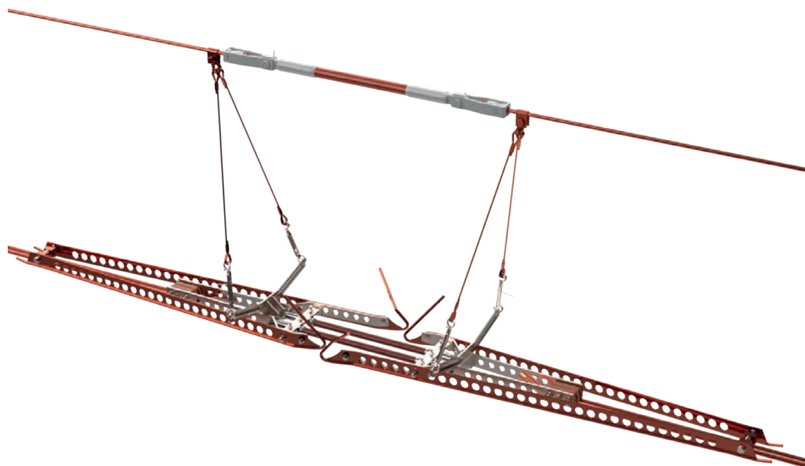
Widok zamontowanego izolatora sekcijnego typu 7520-4
