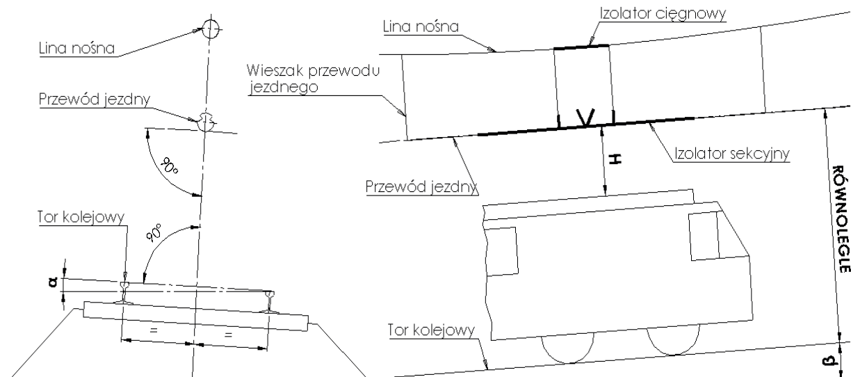
Widok zamontowanego izolatora sekcyjnego typu 7520-3 (7520-4)
