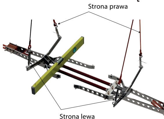
Ustawienie kąta pochylenia poprzecznego \alpha
