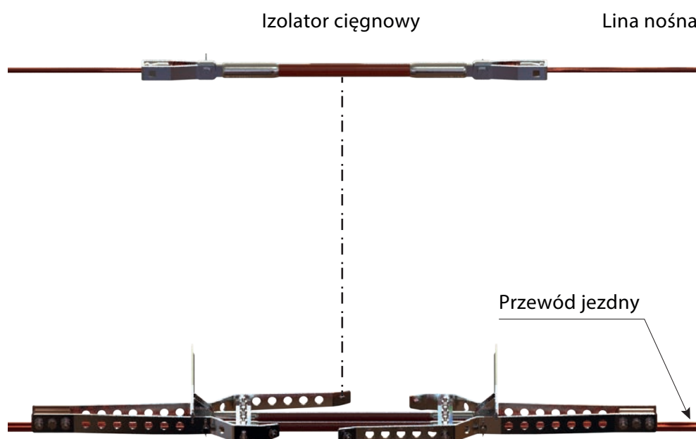
Podzespół nośny izolatora sekcijnego 7520-3 (7520-4)
